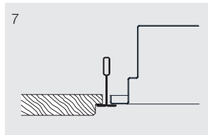
7 Pannelli in fibra minerale con decoro in rilievo 600x600.
