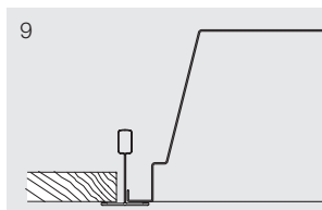
9 Pannelli in fibra minerale 600x600, 600x1200 con struttura in vista.
