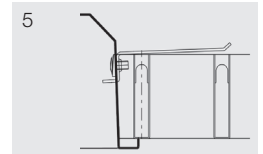
5 Installazione in battuta su controsoffitti grigliati. Apparecchi a richiesta, installati in battuta con staffe accessorie 15 ZH.
